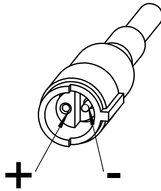
Buchse Receptacle
