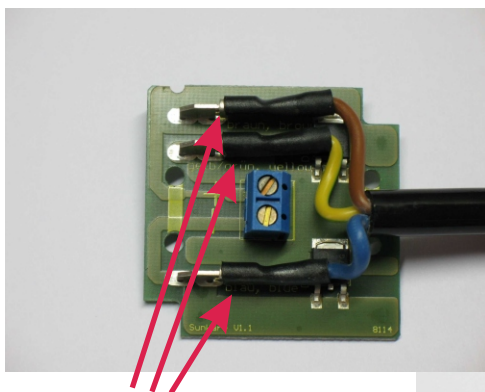
Aufstecken der Kabel
